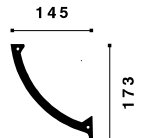
L3 ARSTYL® 173 x 145 x 2000 mm
